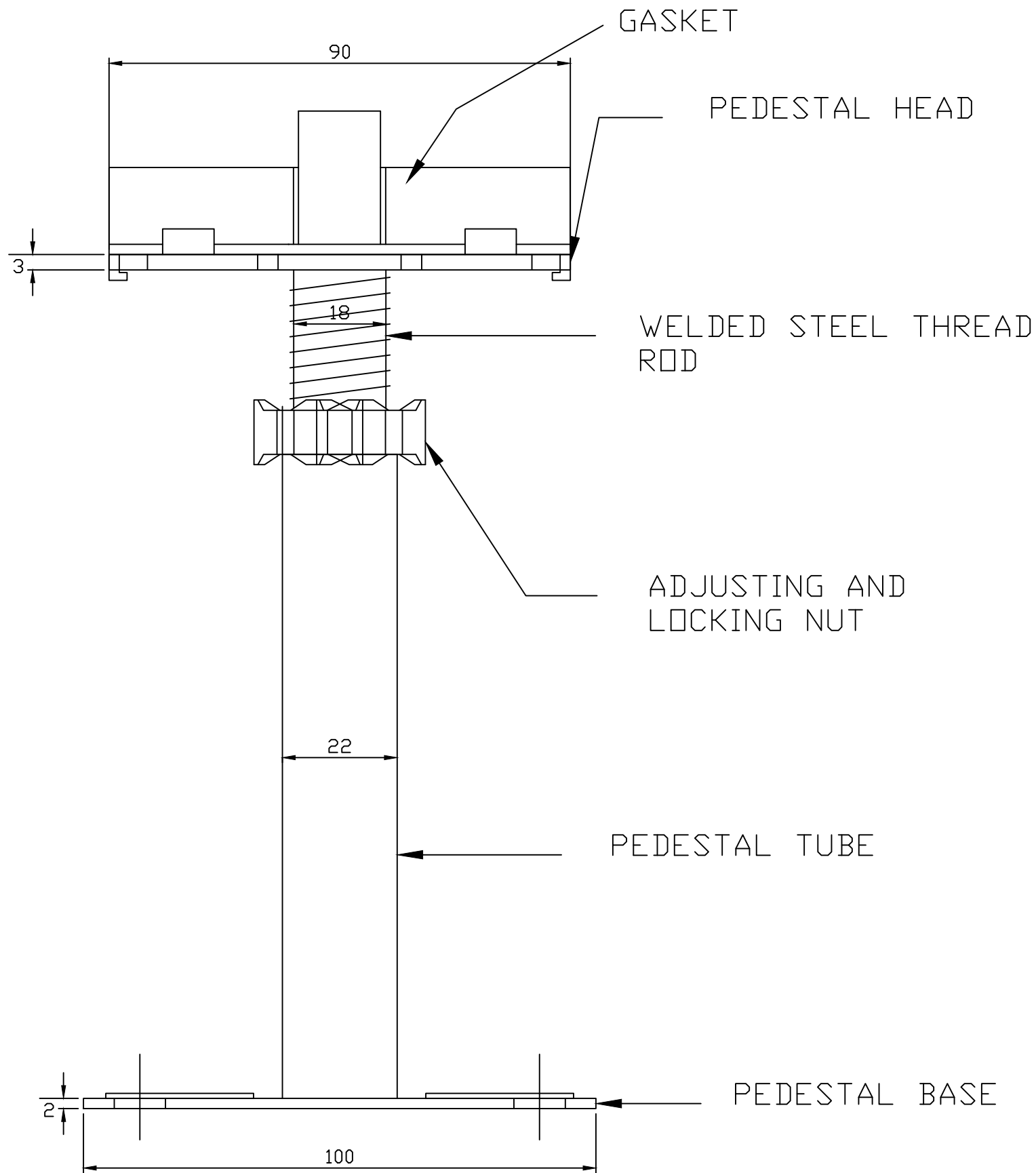
Elevation
