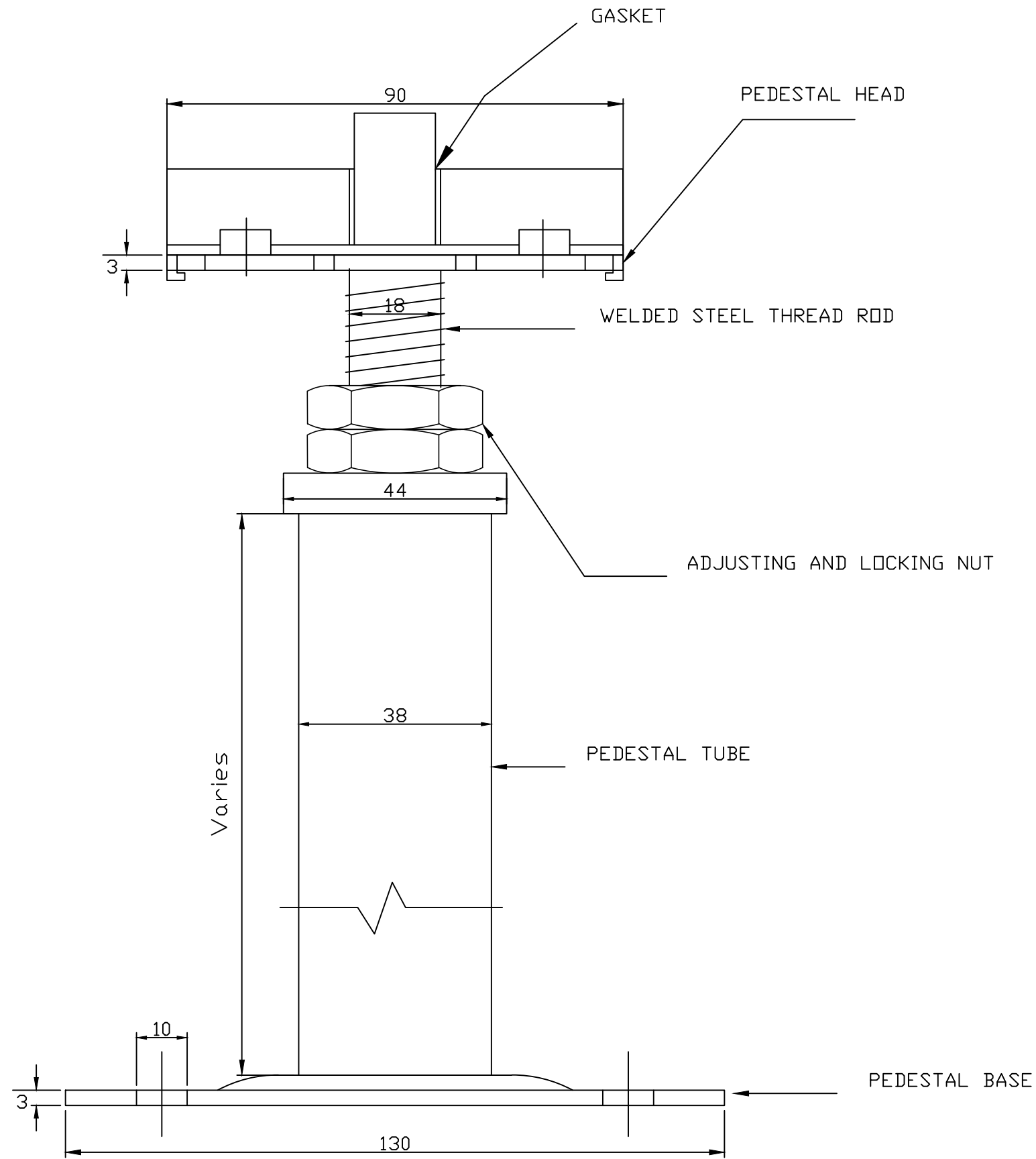
Elevation
